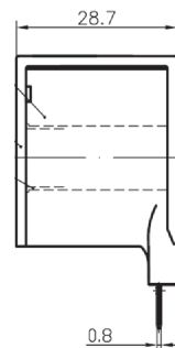
Spulen mit Flachsteckeranschlüssen (SQ-A47 and SQ-D44 Series)
