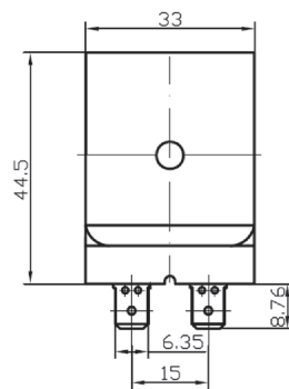
Spulen mit Flachsteckeranschlüssen (SQ-A47 and SQ-D44 Series)
