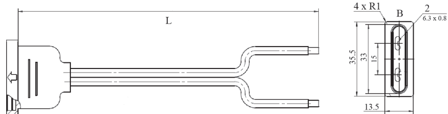
Kabelsatz für Spulen mit Flachstecker (SQ-000000-0900xx)
